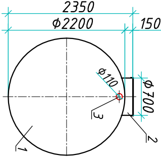
Вид А
